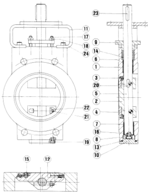
Dettagli costruttivi
