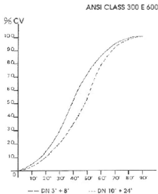
Coefficienti di flusso "CV con valvola aperta a 90° "CV" flow coefficient with valve open at 90°
